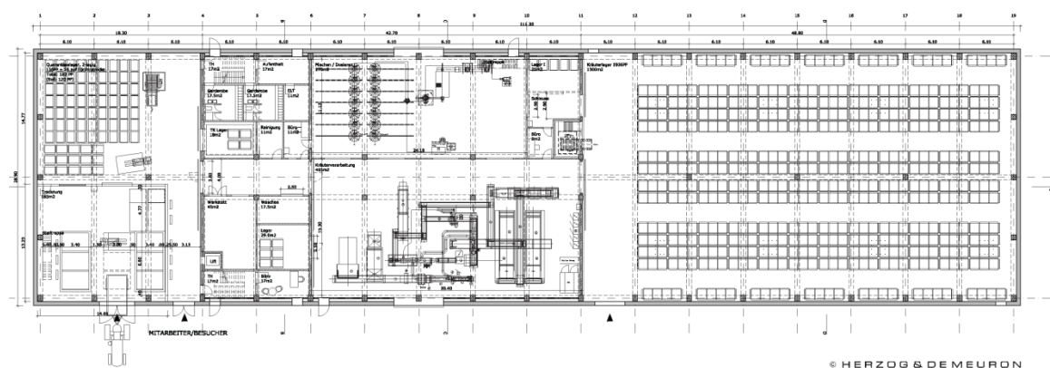
Abb.2: Grundriss Erdgeschoss
