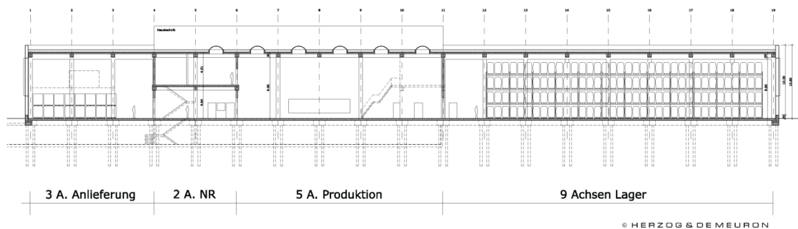
Abb.1: Schnitt Längsachse
